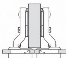
Ușă semiaplicată
