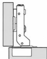
Ușă semiaplicată
